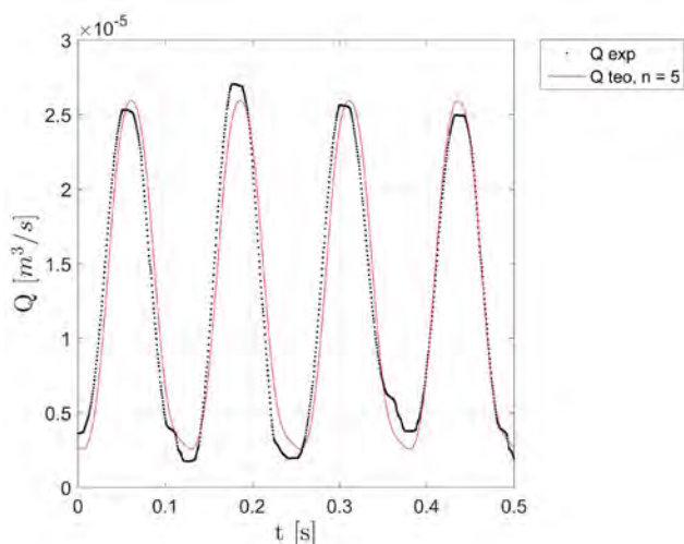
Figura 4. Validación global del modelo. La línea roja representa la predicción teórica, y la línea punteada negra los datos experimentales
