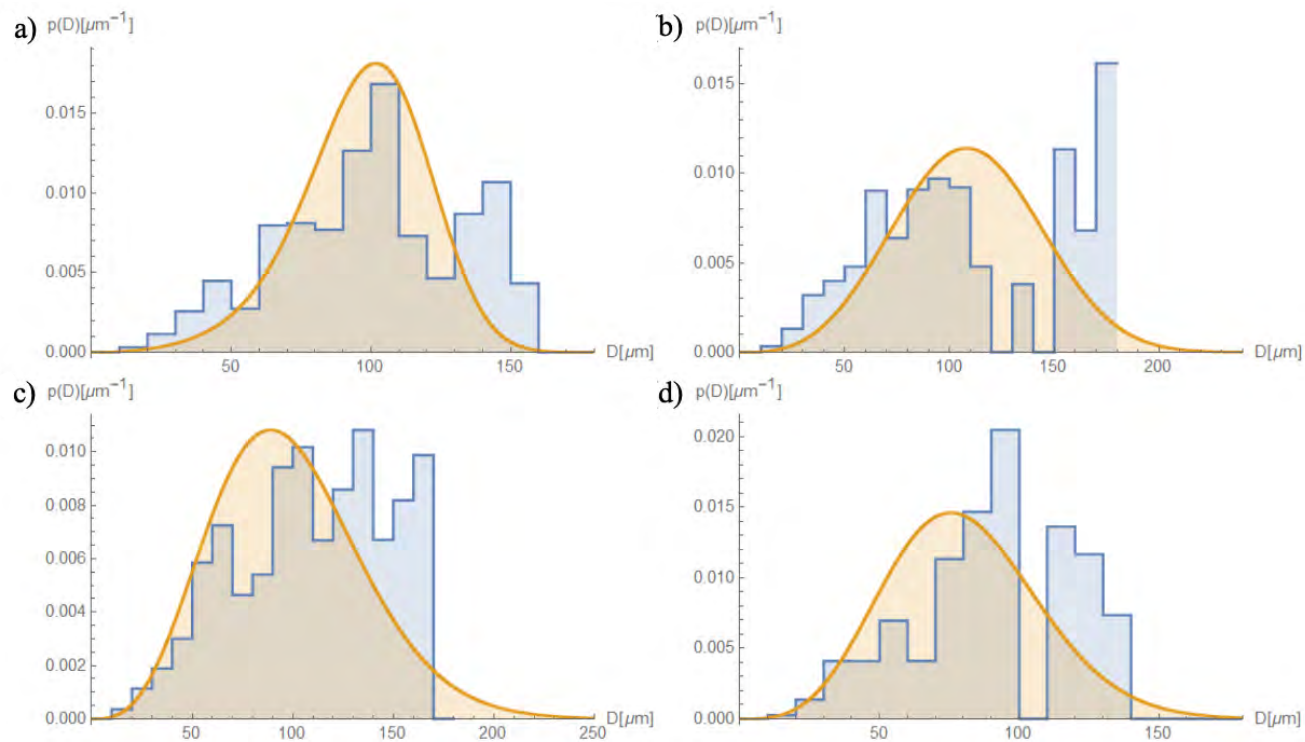
Figura 2. Comparación de las distribuciones calculadas, de color naranja, con las experimentales, de color azul para atomización de agua a) frecuencia de 40 kHz, desplazamiento de 4.5 \mu\text{m} y gasto de 10 cc/min, b) 40 kHz, 7 \mu\text{m} y 30 cc/min, c) 60 kHz, 4.7 \mu\text{m} y 20 cc/min, d) 70 kHz, 3.9 \mu\text{m} y 20 cc/min
