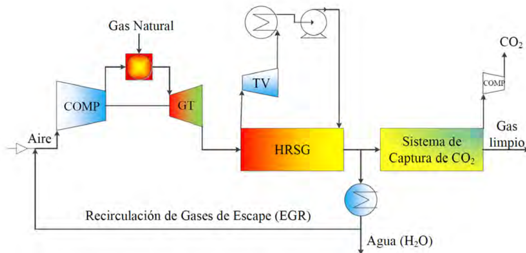
Figura 2. Diagrama simplificado de una NGCC con recirculación de gases de combustión y captura de \text{CO}_2 , elaboración propia a partir de Merkel et al. (2013)
