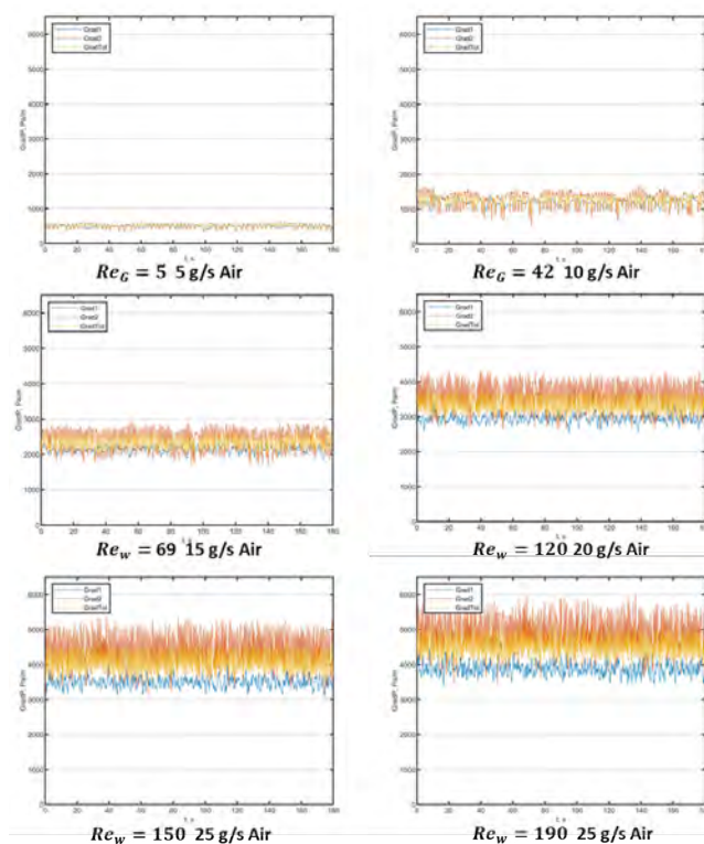
Figura 3. Señales típicas de experimentos bifásicos líquido-gas en patrón de flujo intermitente
