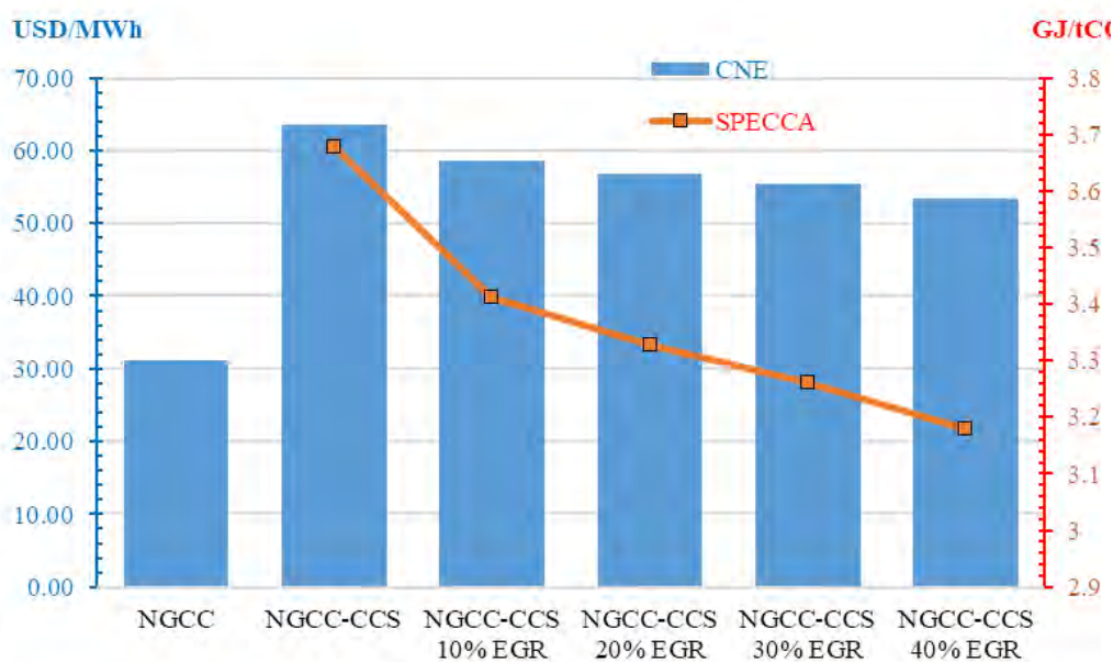
Figura 3. Comparativa del incremento de CNE para el sistema NGCC con captura de \text{CO}_2 y sistema EGR con SPECCA, elaboración propia
