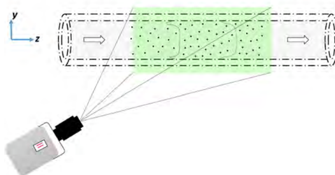
Figura 3. Método de iluminación con una hoja láser
