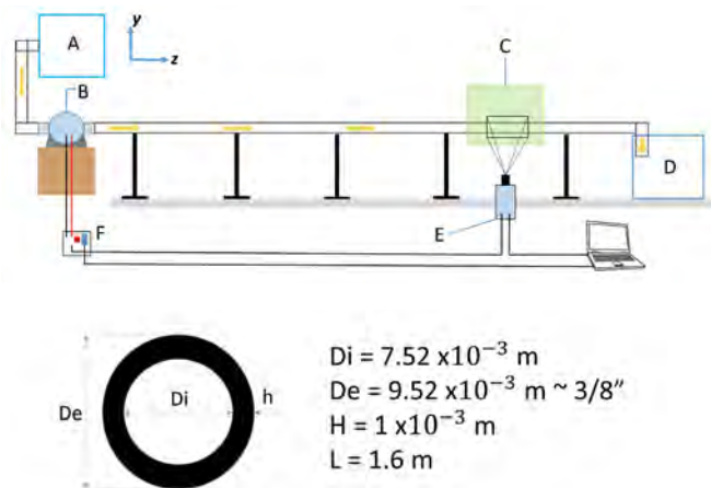
Figura 2. Arreglo experimental A: Depósito de alimentación, B: Bomba peristáltica, C: Hoja láser, D: Depósito de descarga, E: Cámara de alta velocidad, F: Circuito de control
