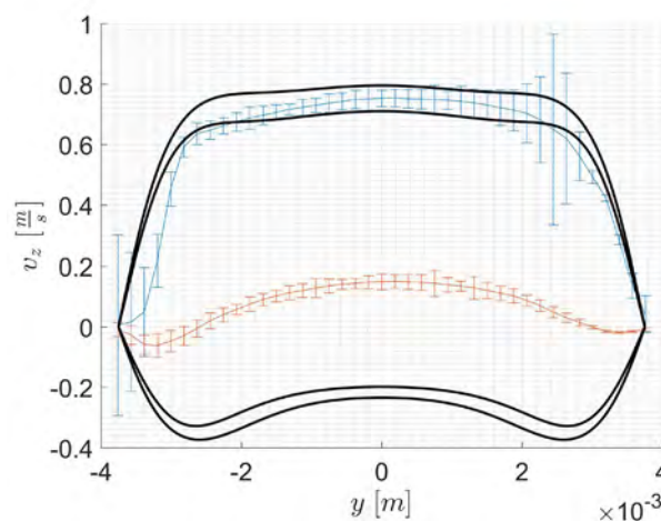
Figura 5. Validación local. El perfil de velocidades en la fase impulsiva se compara favorablemente con la predicción teórica. En la fase de retroceso del flujo se produce un desfase del perfil, probablemente ocasionado por limitaciones asociadas a la técnica PIV
